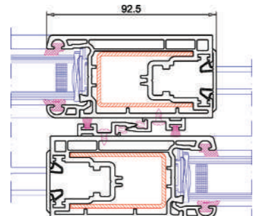
Sección central puerta
